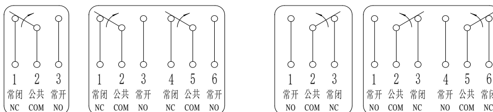
图 2 三芯常开常闭接点、六芯双常开常闭接点压力释放阀接线原理图
