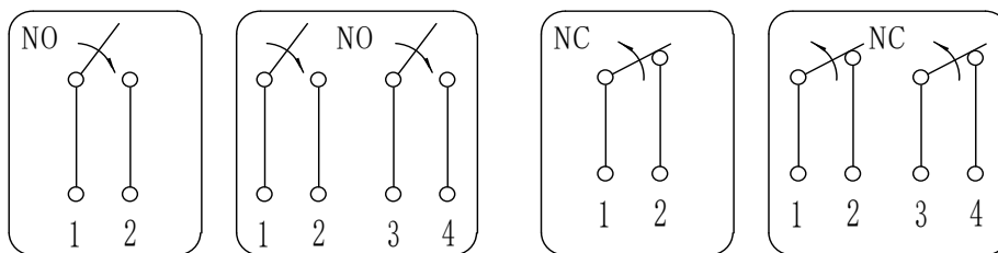
图 1 二芯常开 (常闭) 接点、四芯双常开 (常闭) 接点压力释放阀接线原理图
